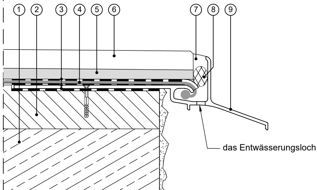
das Detail A
